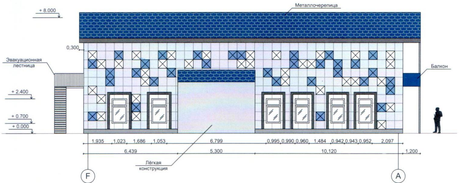
Проект. Схема фасада
